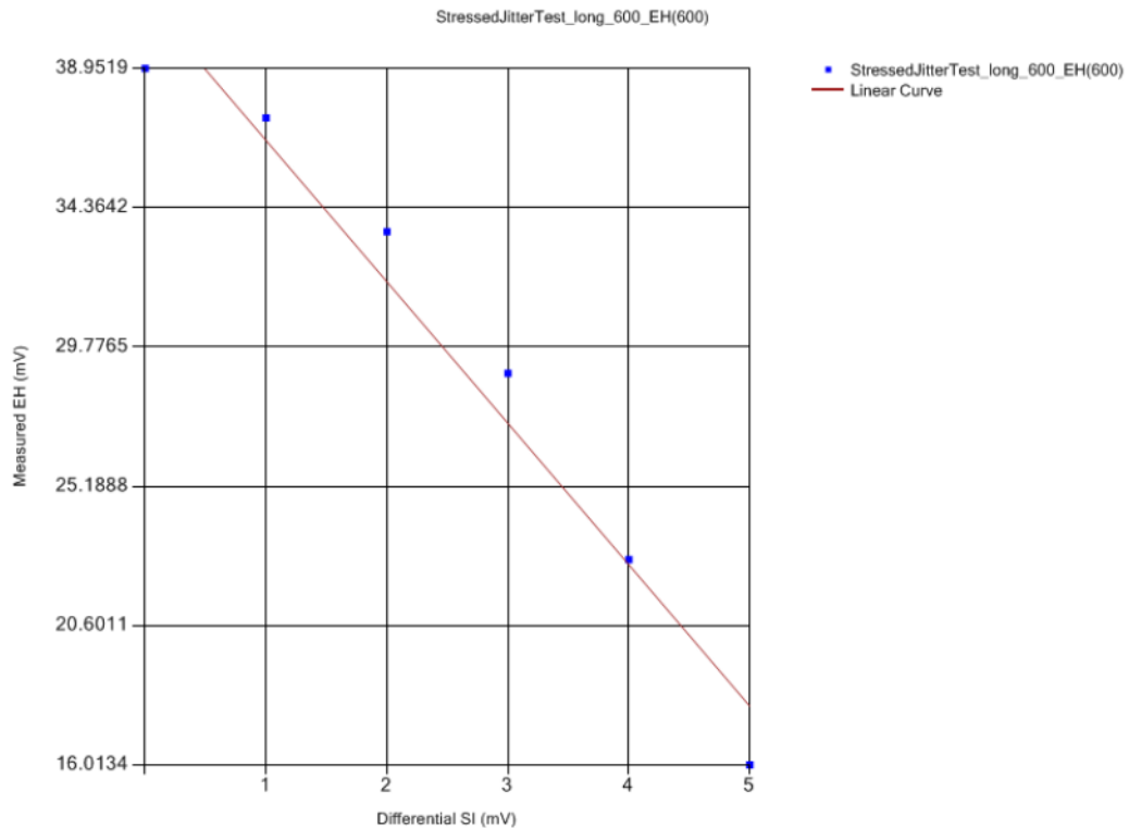
StressedJitterTest_long_600_EH(600) Plot
