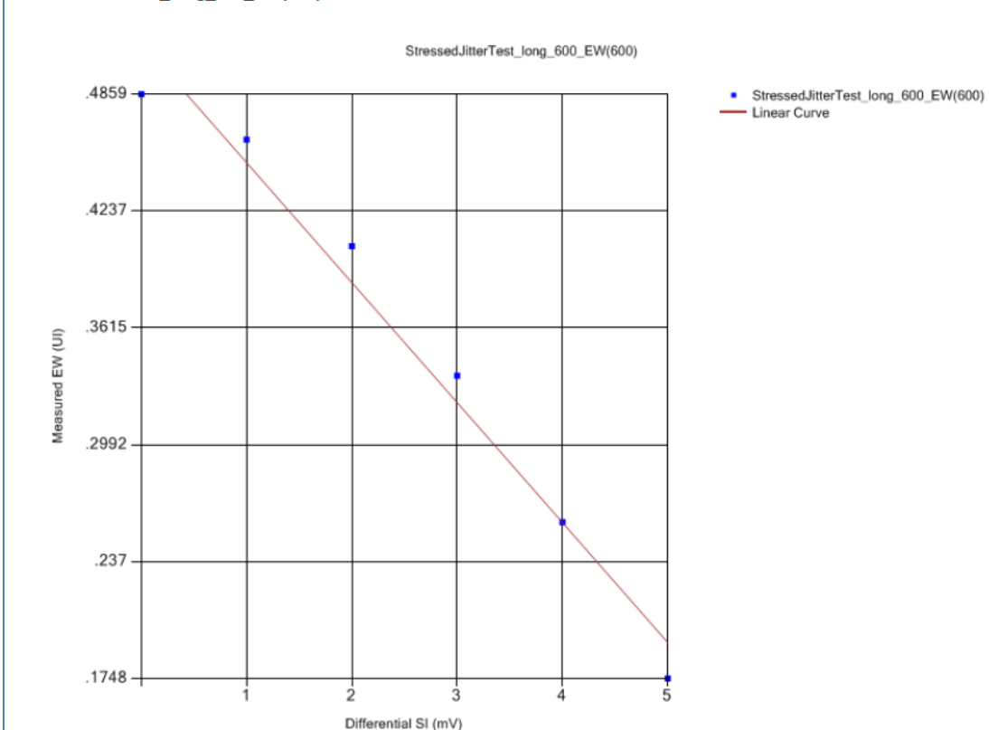
StressedJitterTest_long_600_EW(600) Plot
