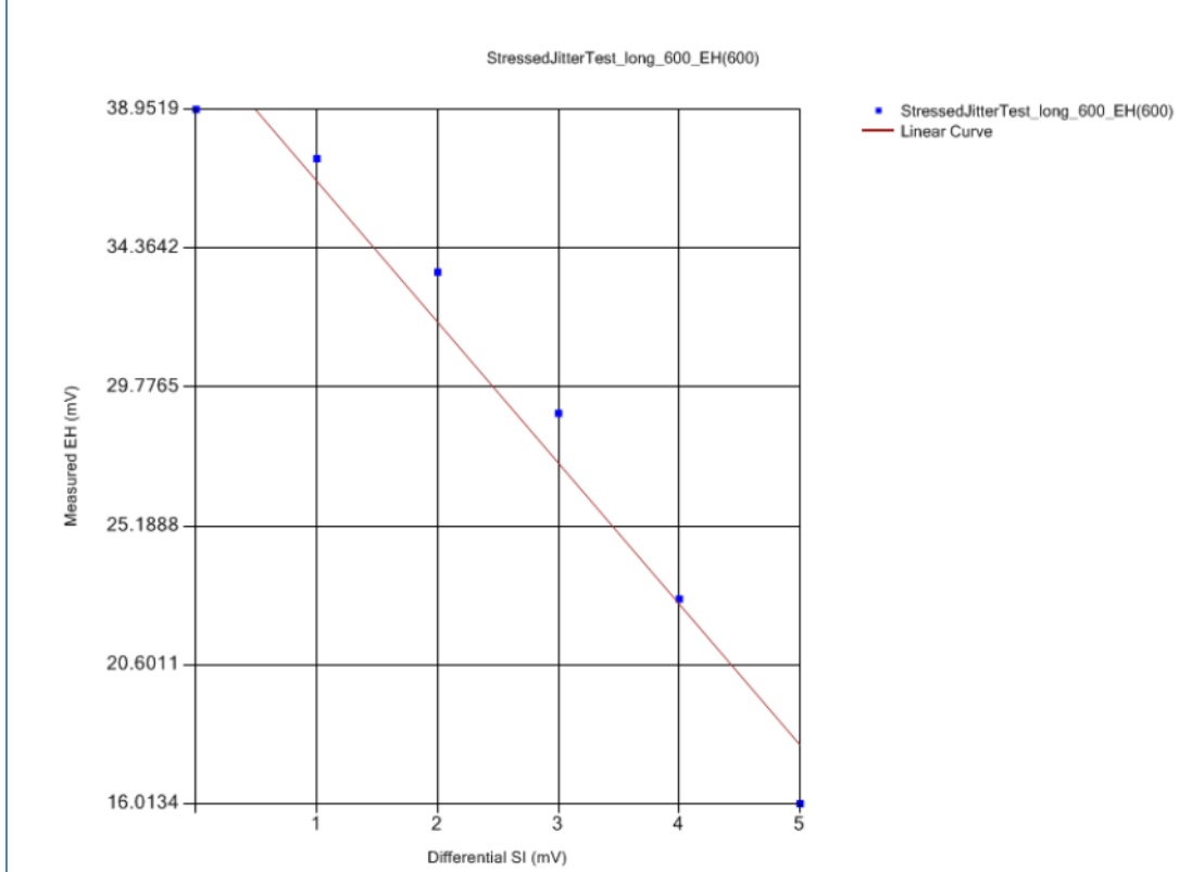
StressedJitterTest_long_600_EH(600) Plot
